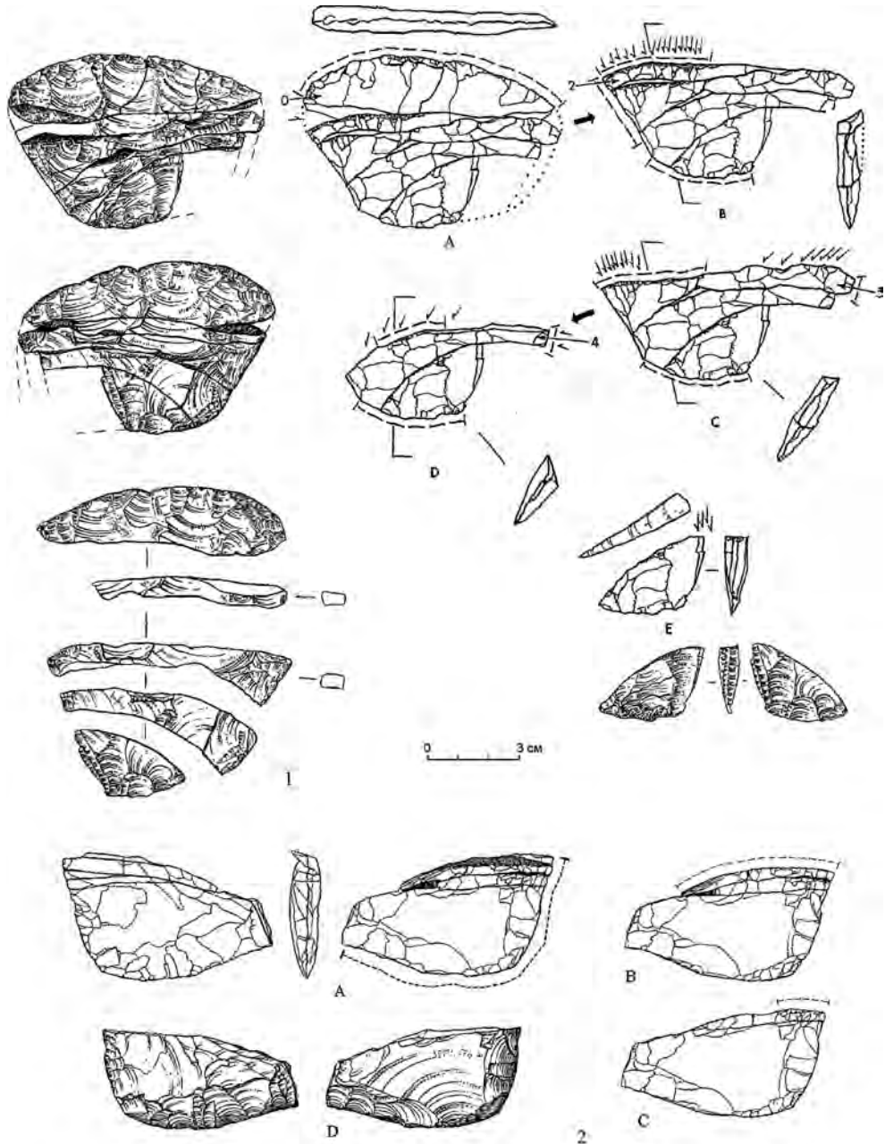
Рис. 5. Большой Якорь I, сборки бифасов из культурного горизонта 7. 1 — бифас на различных этапах переоформления (А, В, С, D) с переходом в микронуклеус; 2 — бифас на различных этапах переоформления (А, В, С, D) с функциями ножа и скребла (по: Инешин, Тетенькин 2010: рис. 6.11) Fig. 5. Bol'shoi Yakor' I. Conjoined bifaces from cultural horizon 7. 1 — biface at various stages of reshaping (A, B, C, D), ending with a microcore stage; 2 — biface at various stages of reshaping (A, B, C, D), combining the functions of knife and scraper (after: Ineshin, Tetenkin 2010: fig. 6.11)
