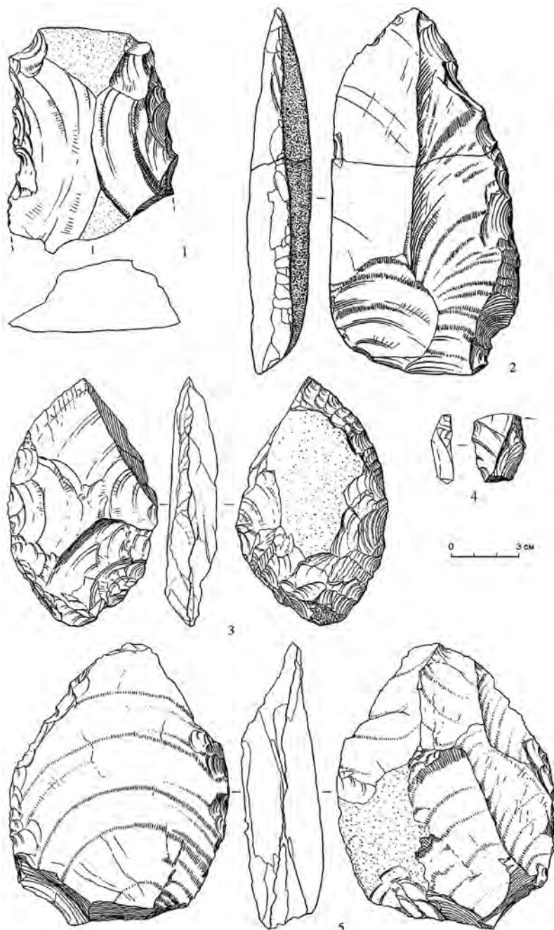
Рис. 6. Большой Якорь I, изделия из культурного горизонта 5. 1, 2, 5 — унифасиальные орудия (скрёбла); 3 — бифас-нож; 4 — трансверсальный резец (по: Инешин, Тетенькин 2010: рис. 6.50) Fig. 6. Bol'shoi Yakor' I. Artifacts from cultural horizon 5. 1, 2, 5 — unifacial tools (end-scraper); 3 — biface-knife; 4 — transversal burin (after: Ineshin, Tetenkin 2010: fig. 6.50)
