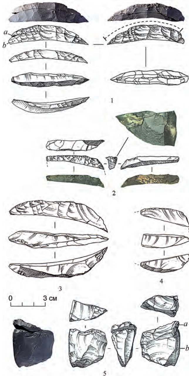
Рис. 11. Коврижка IV, изделия из камня: 1 — ребёрчатый (a) и лыжевидный (b) сколы; 2–4 — лыжевидные сколы; 5 — нуклеус (a) и апплицированная к нему ударная площадка (b) (1 — к. г. 2Б; 2 — к. г. 3Б; 3 — к. г. 4; 4 — к. г. 5; 5 — к. г. 6). 1, 3–5 — по: Тетенькин 2017
