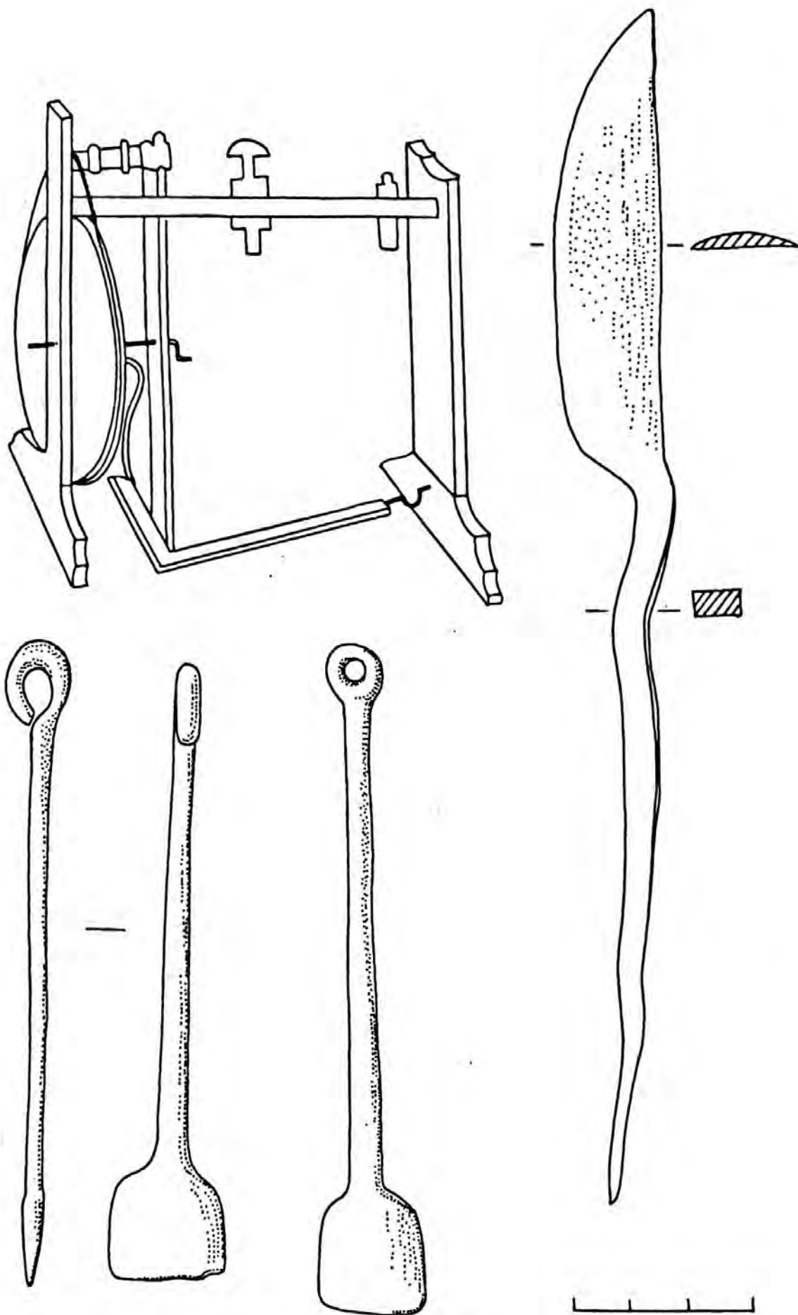
Рис. 12. Крестьянский токарный станок XIX в. Железные инструменты (костерезы)
