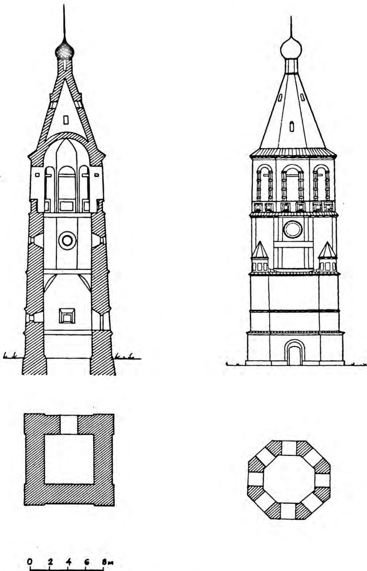
Рис. 27. Холмогоры. Колокольня. Восточный фасад, разрез и планы этажей
