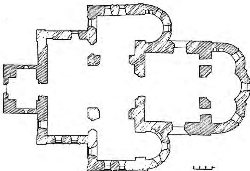
Рис. 32. Верхние (Никольские) Матигоры. Храм Николая Чудотворца (пересвящен в Вознесенскую). Южный фасад и план
