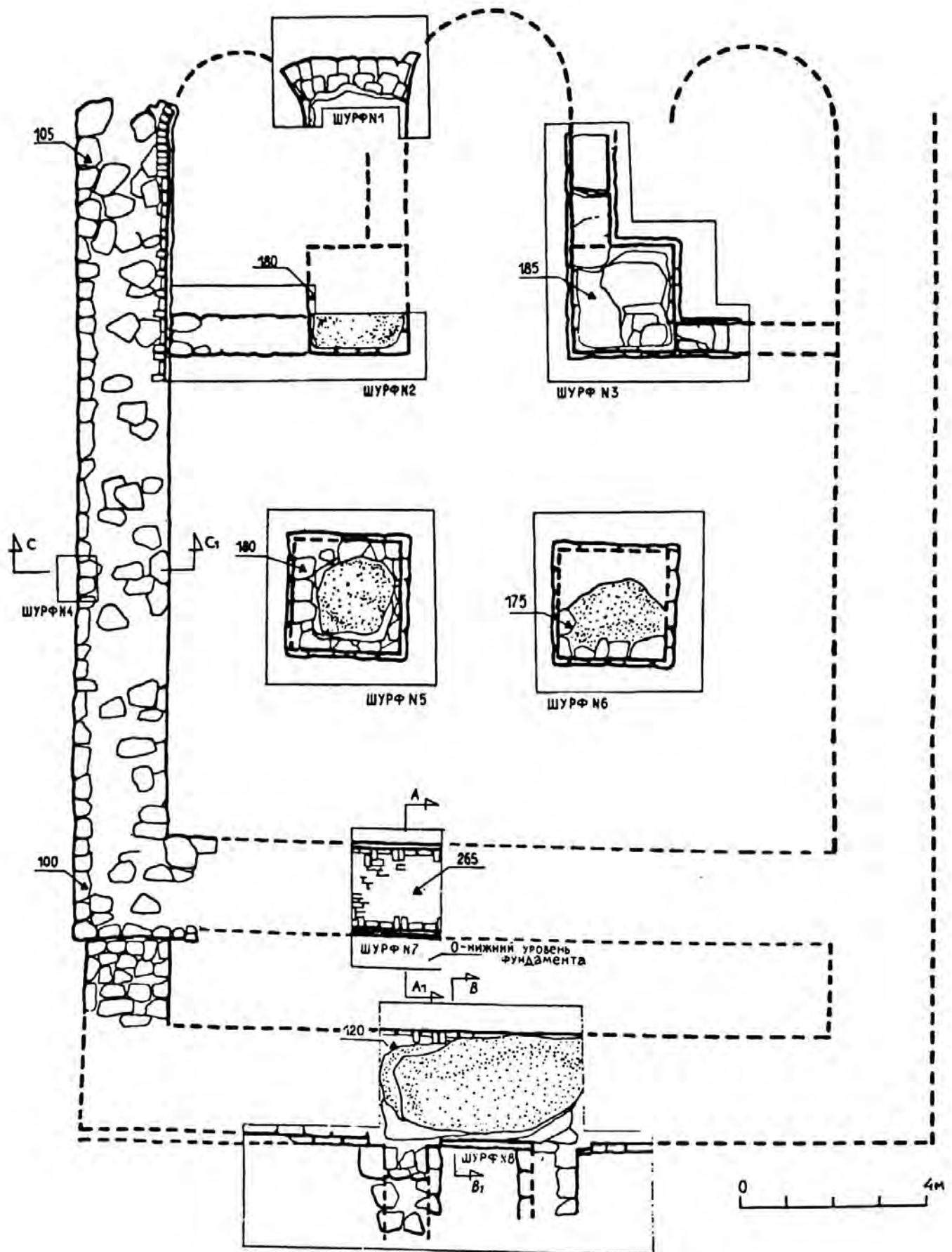
Рис. 21. Нижние Матигоры. Храм св. мучеников Бориса и Глеба. План здания по материалам архитектурно-археологического исследования
