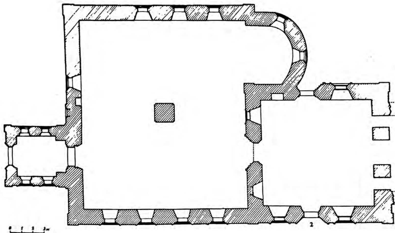
Рис. 48. Кур-остров. Церковь Великомученика Дмитрия Солунского. Обмер 1975 г. 1 — южный фасад, 2 — план
