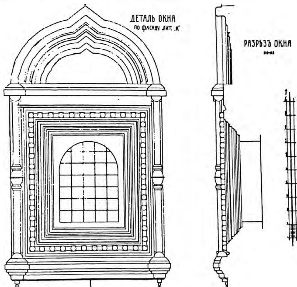
Рис. 40. Ухт-остров. Троицкий собор. Деталь окна. Обмер 1912 г.
