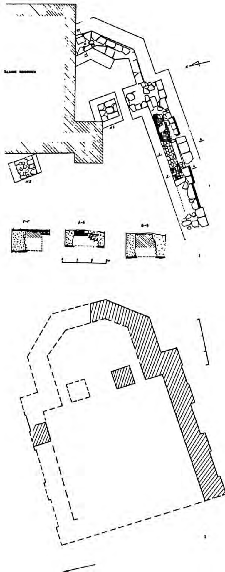
Рис. 51. Деревня Вавчуга. Церковь Иоанна Предчети. 1 — фрагмент плана церкви (архитектурно-археологические исследования 1975 г.), 2 — реконструкция основного объема здания. Фрагмент
