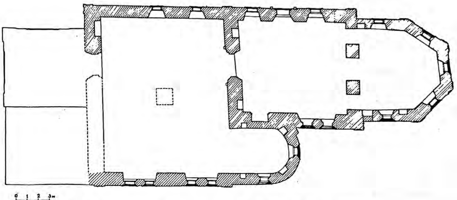
Рис. 47. Красногорский Пинежский монастырь. Храм Похвалы Пресвятой Богородицы. План. Обмер 1976 г.
