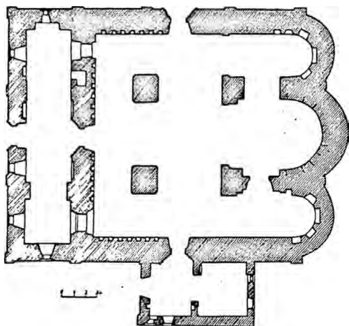
Рис. 4. Антониев-Сийский монастырь. Троицкий собор. План. Обмер 1975 г.
