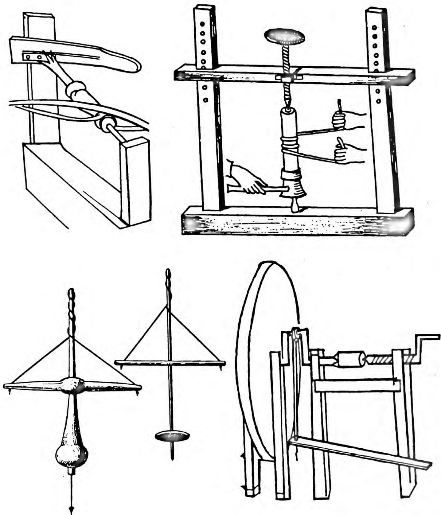
Рис. 13. Европейские токарные станки XIV—XVII вв.
