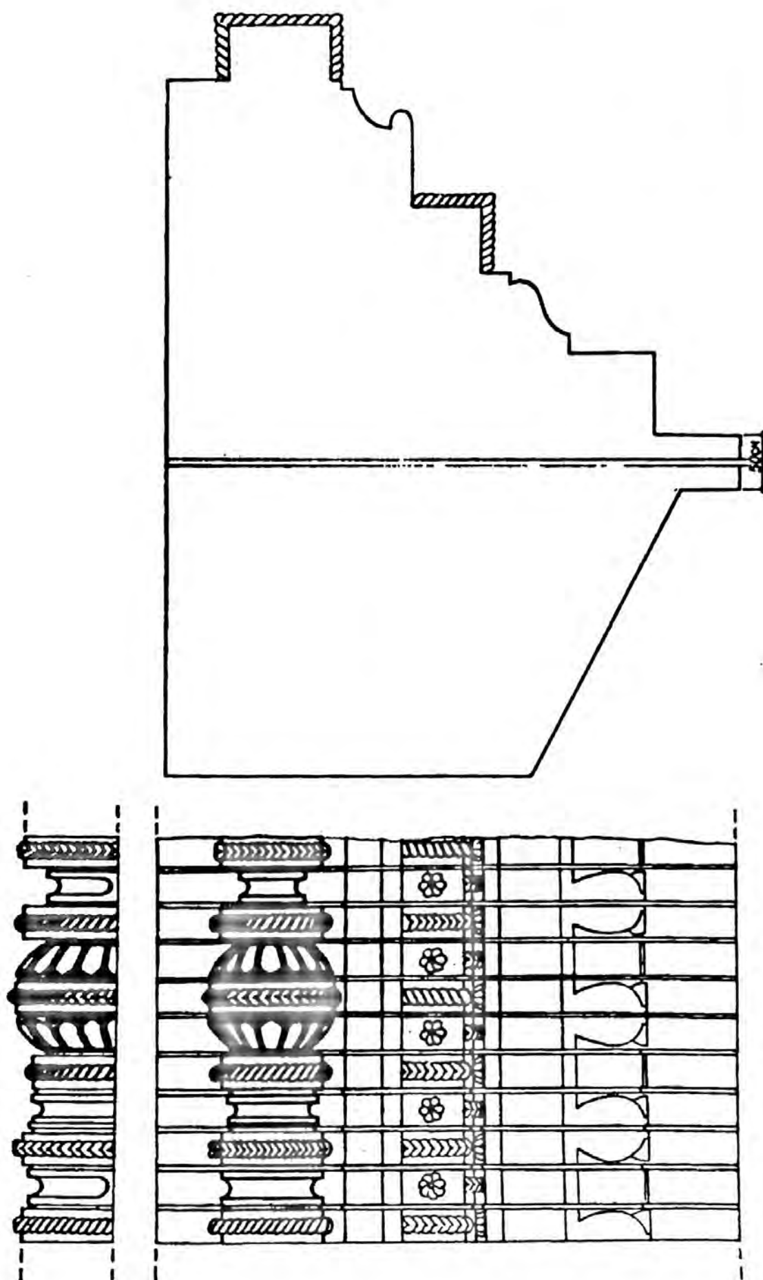
Рис. 17. Спасо-Прилуцкий Козьмеручьевский монастырь. Собор Спаса Нерукотворного. Деталь западного портала. План и профиль
