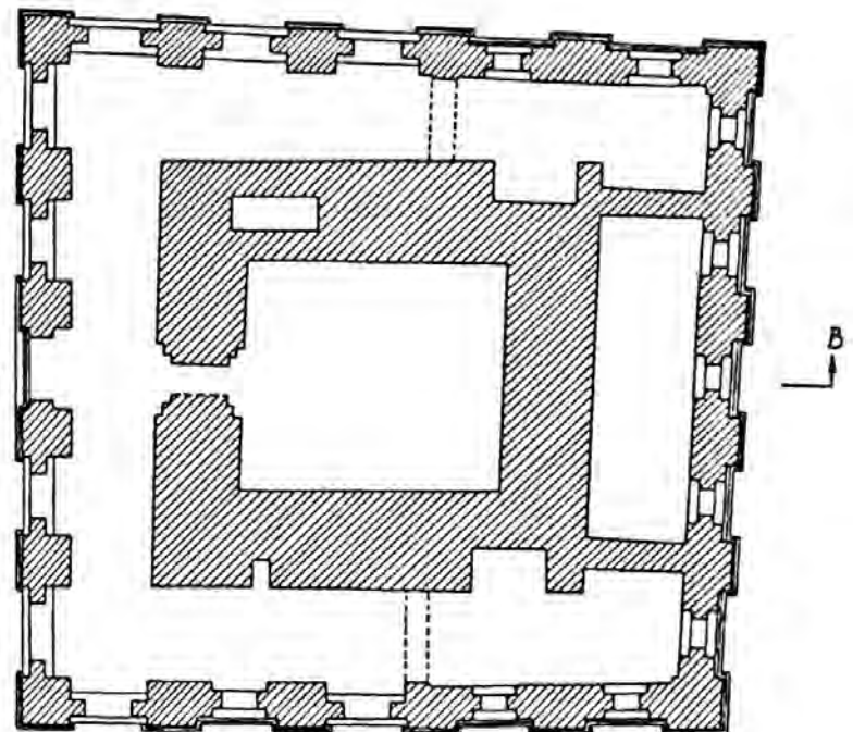
План 2 го этажа
