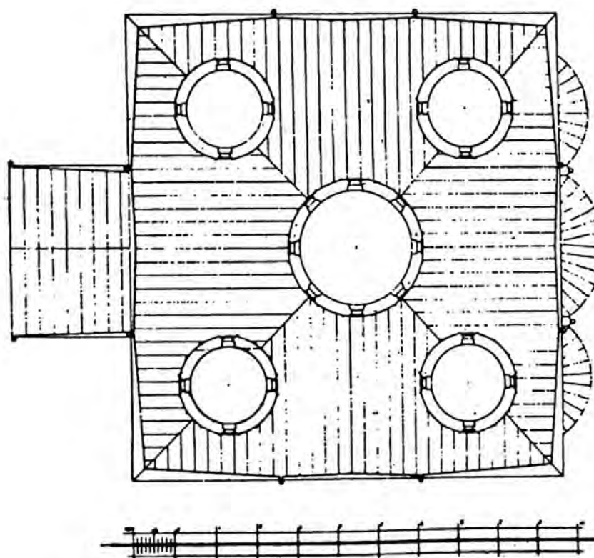
Рис. 38. Ухт-остров. Троицкий собор. План собора и крыши. Обмер 1912 г.
