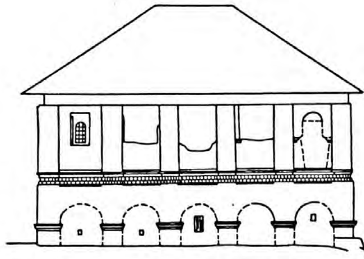
СЕВЕРНЫЙ ФАСАД
