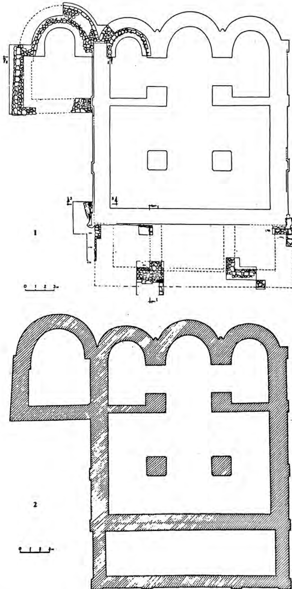
Рис. 42. Ухт-остров. Троицкий собор. 1 — план по данным архитектурно-археологических работ, 2 — реконструкция планов церкви и придела
