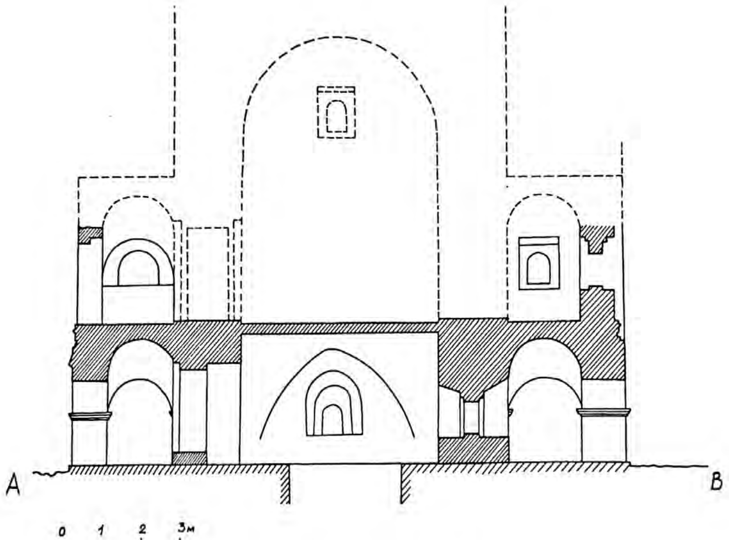
Разрез здания по линии север-юг
