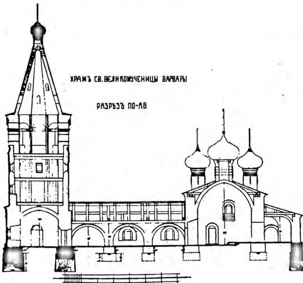
Рис. 44. Ухт-остров. Церковь Великомученицы Варвары. Южный фасад и продольный разрез церкви
