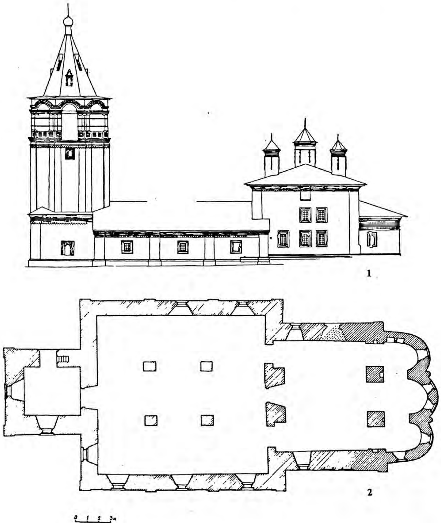
Рис. 46. Ухт-остров. Церковь Великомученицы Варвары. Обмер 1975 г. 1 — южный фасад храма, 2 — план
