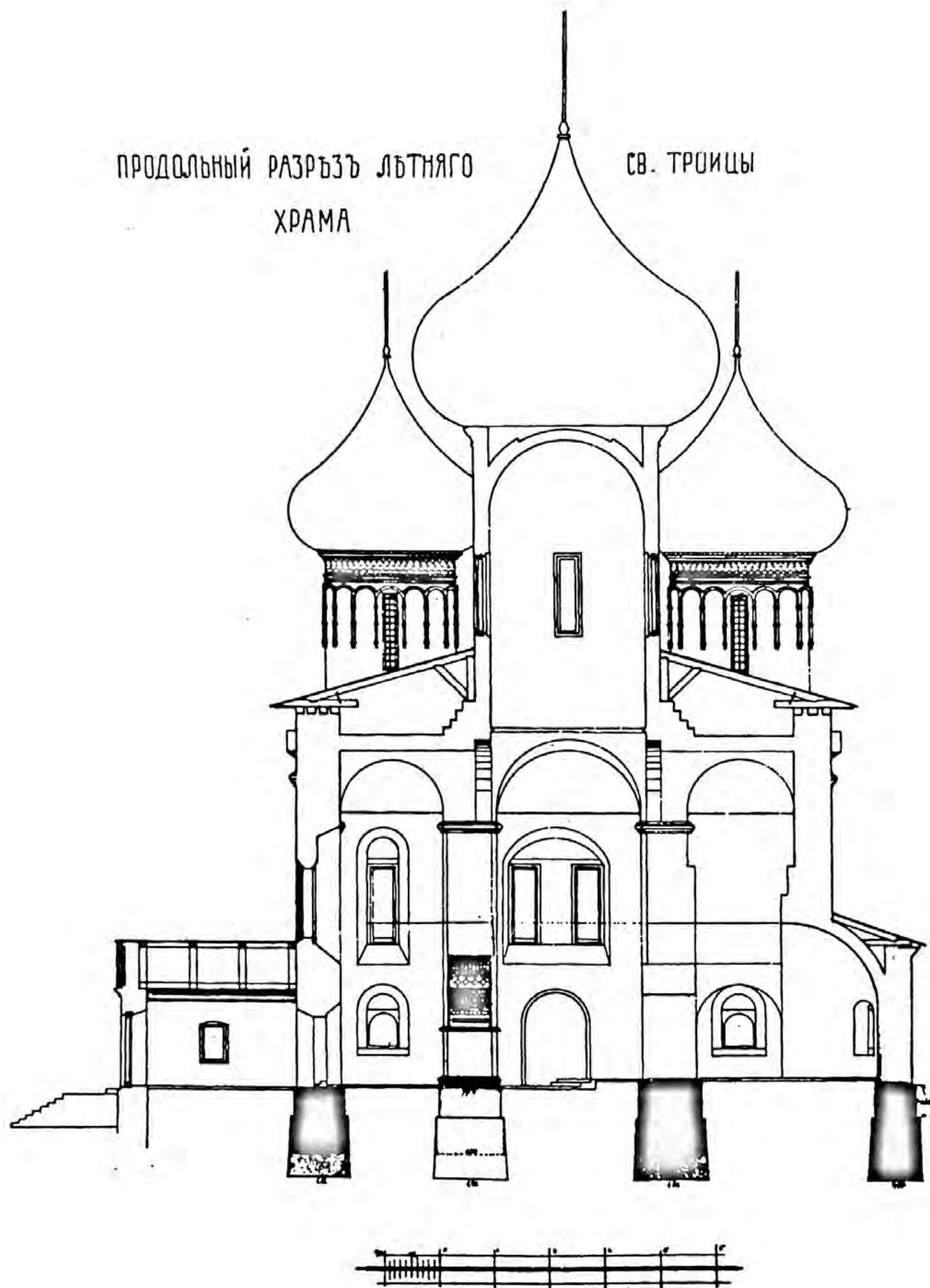
Рис. 37. Ухт-остров. Продольный разрез Троицкого собора. Обмер 1912 г.
