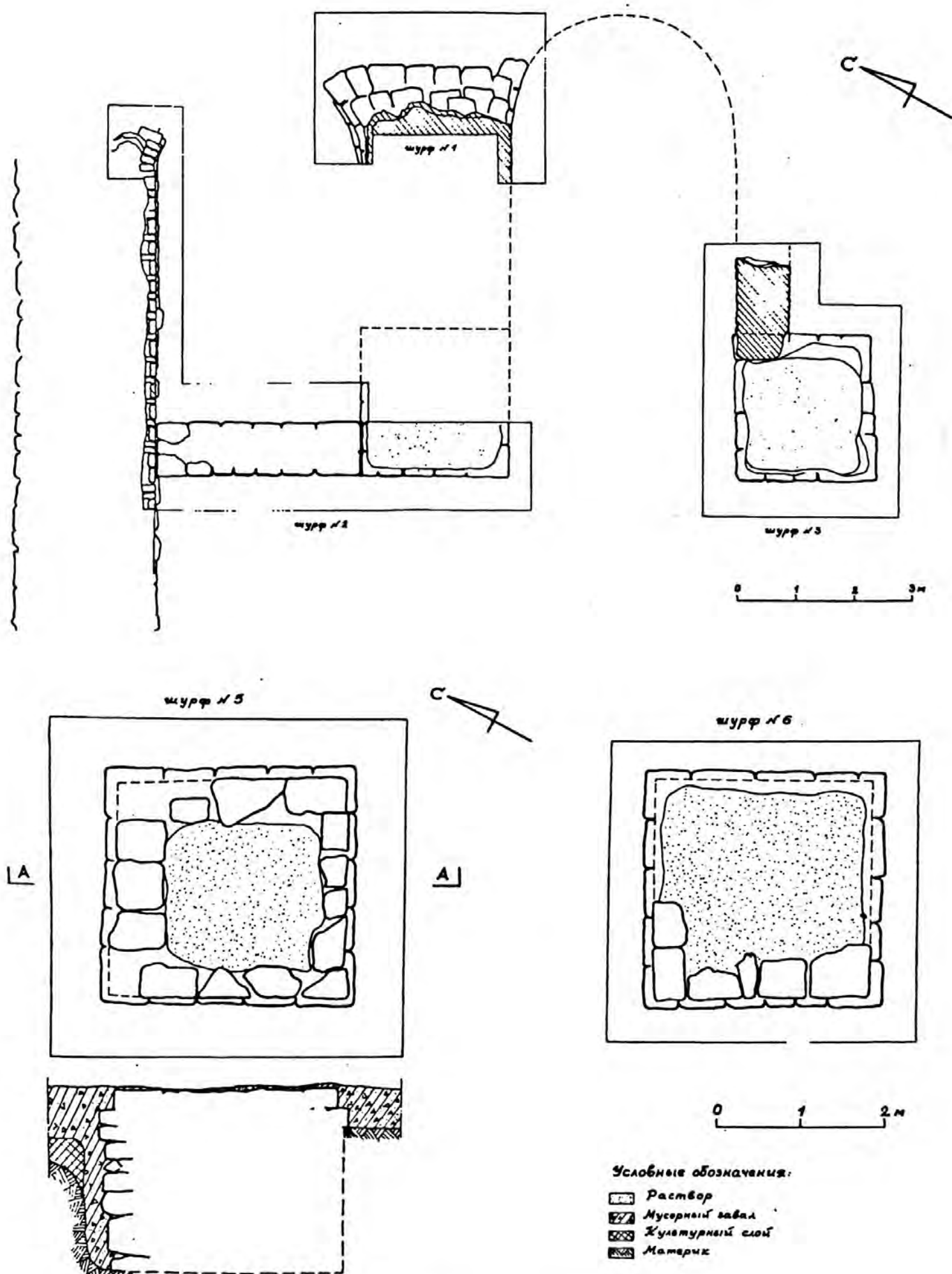
Рис. 22. Нижние Матигоры. Храм св. мучеников Бориса и Глеба. Планы и разрезы шурфов
