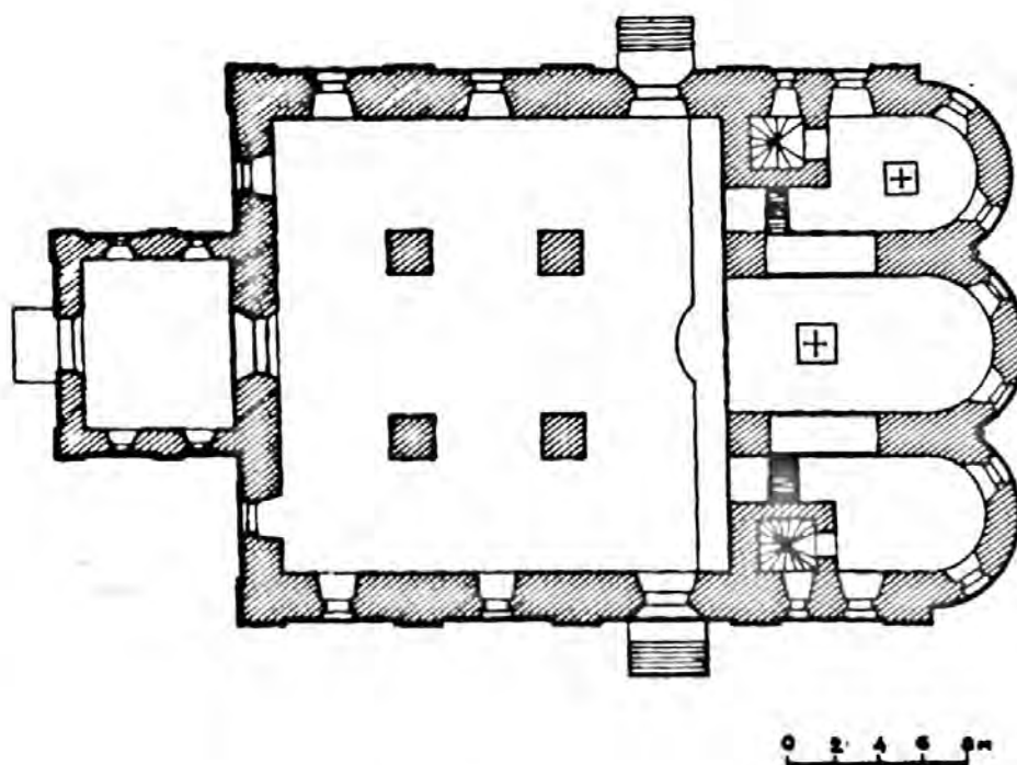
Рис. 28. Холмогоры. Спасо-Преображенский собор. Южный фасад и план
