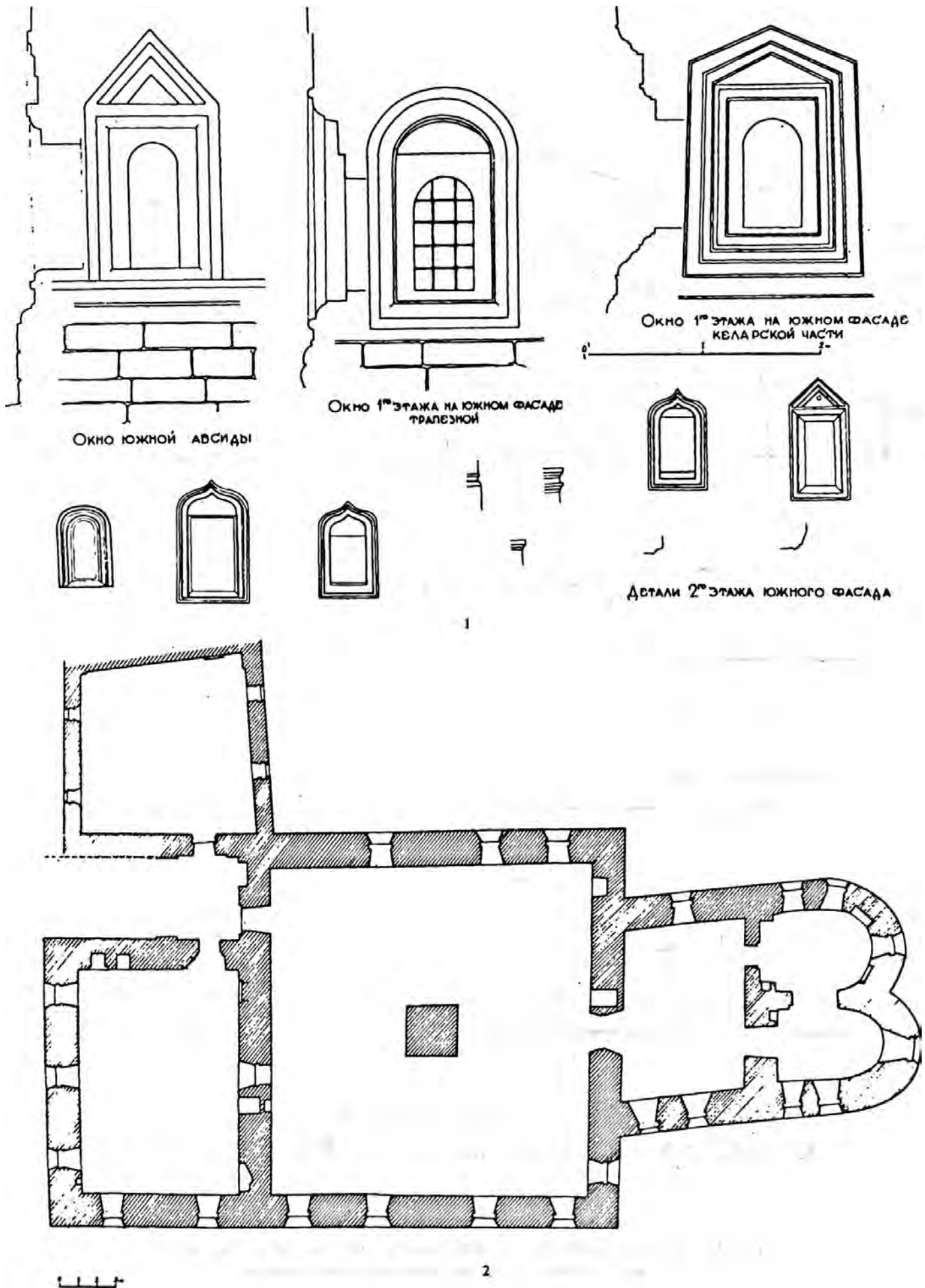
Рис. 10. Антониев-Сийский монастырь. Благовещенская церковь. 1 — детали южного фасада, 2 — план церкви, трапезной и келарской
