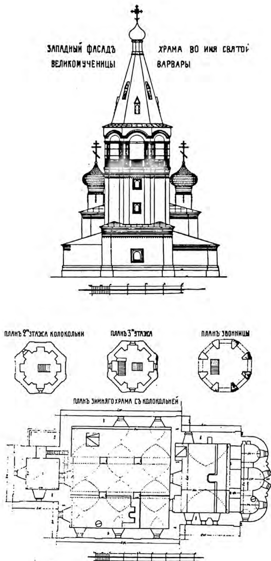
Рис. 45. Ухт-остров. Церковь Великомученицы Варвары. Западный фасад, план церкви и ярусов колокольни. Обмер 1912 г.
