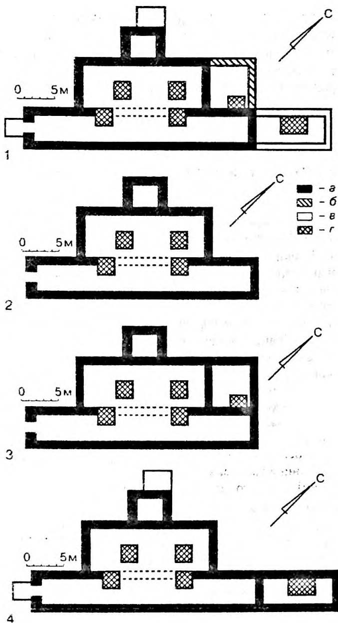
Рис. 11. Строительная история постройки № 1 (по результатам раскопок 1999 г.): 1 — стратиграфия кладок XIX в.; 2 — первый строительный период; 2 — второй строительный период; 4 — третий строительный период; а — кладка на известковом растворе; б—в — кладки на цементном растворе; г — местоположение печей.
