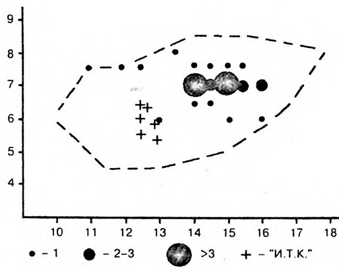
Рис. 8. Параметры кирпичей из раскопок 1999 г.: А — соотношение ширины и толщины (по всем обмерянным кирпичам); Б — соотношение ширины и толщины кирпичей из кладки конца XVIII в. и с клеймом "И. Т. К."
