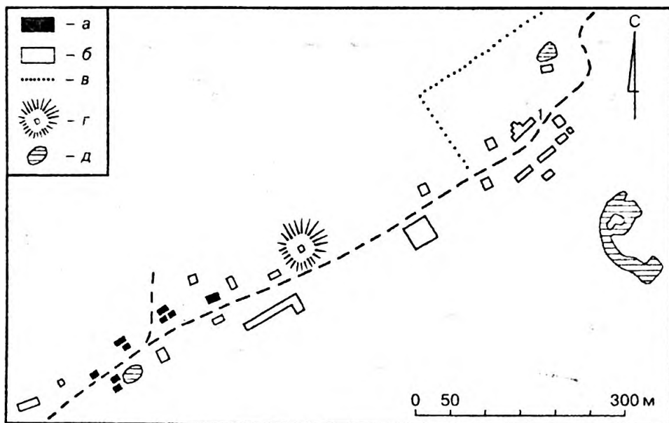
Рис. 2. Схема застройки д. Воскресенское (по топосъемке 1998 г.): а — существующие постройки; б — руинированные постройки и фундаменты построек (1 — постройка, исследованная раскопками 1999 г.); в — границы парка, выявленные при топосъемке; г — горка с остатками фундаментов храма; д — пруды.
