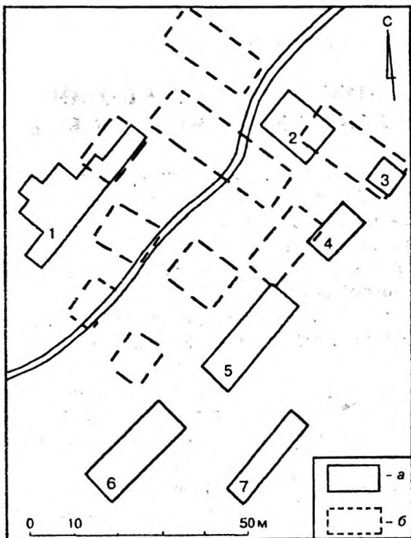
Рис. 15. Совмещение застройки усадьбы Воскресенское конца XVIII в. с современной топосъемкой: а — фундаменты и руины XIX в.; б — предположительное местоположение построек конца XVIII в.
