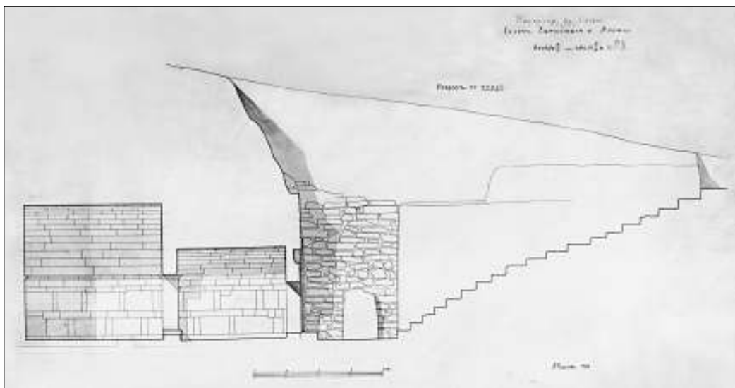
Ольвия. Склеп Евросивия и Ареты (конец II–начало III в. по Р. Х.). Чертеж К. К. Романова 1908 г.
