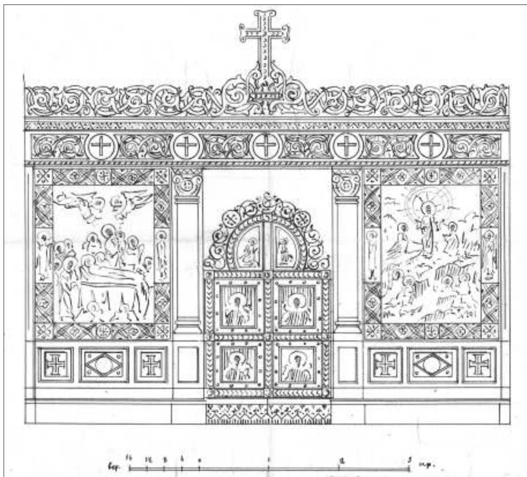
Проект иконостаса Спасского собора Мирожского монастыря выполненный М. Т. Преображенским. 1901 г. (1886 г., д. 63 е, л. 2)
