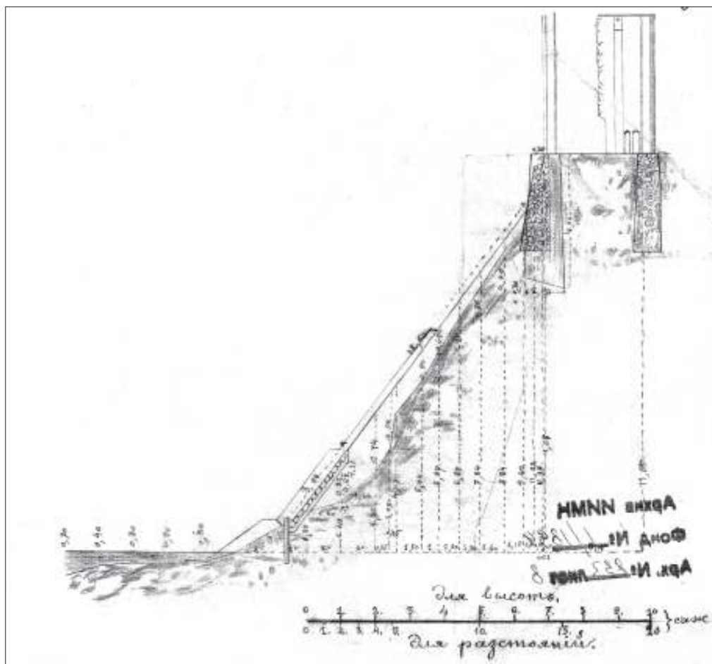
Гродно. Схема устройства укрепляющей площадки под Коложской церковью (1894 г., д. 233, л. 10 об.)
