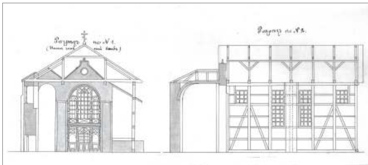
Гродно. Проект деревянного покрытия и стен Коложской церкви (1894 г., д. 233, л. 14)
