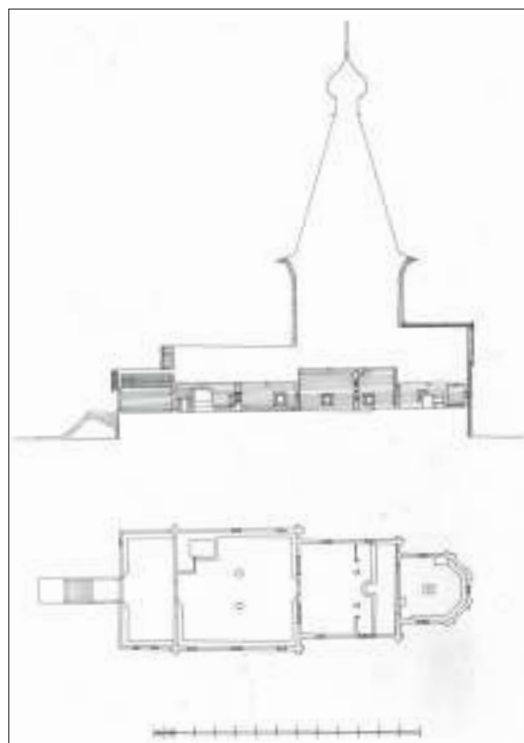
Петропавловская церковь в с. Пучуга Вологодской губернии. Чертежи Д. В. Милеева (ФА, III 9934)
