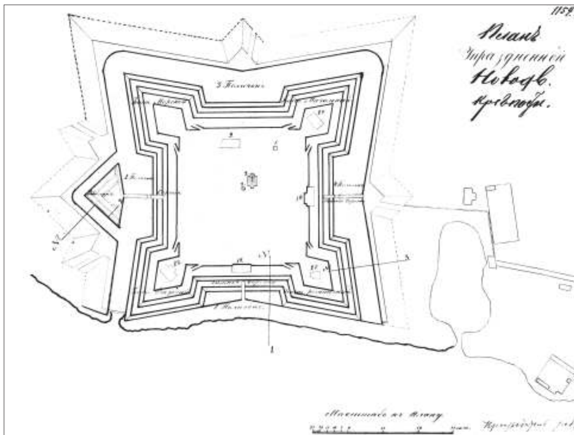
План Новодвинской крепости. Архангельская губерния (1897 г., д. 276, л. 15)
