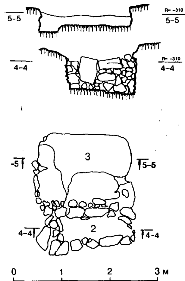
Рис. 6. Планы и разрезы могил 2 и 3
