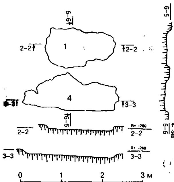
Рис. 5. Планы и разрезы могил 1 и 4
