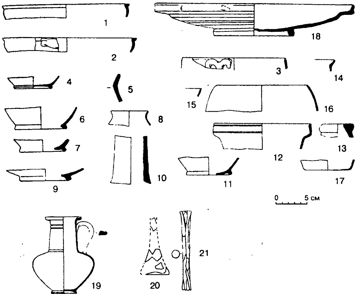
Рис. 3. Керамические и стеклянные сосуды из могильника
