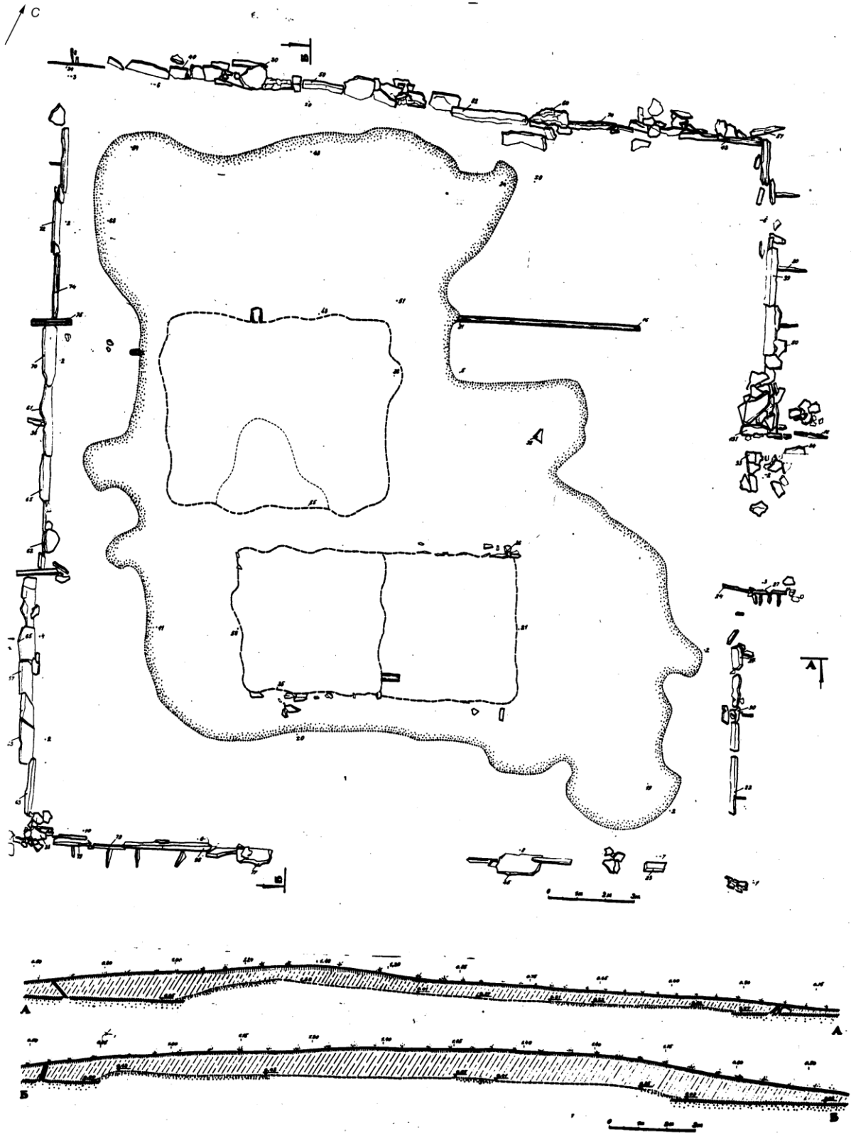
4. Курган Береш III. План подкурганых сооружений. Разрезы.
