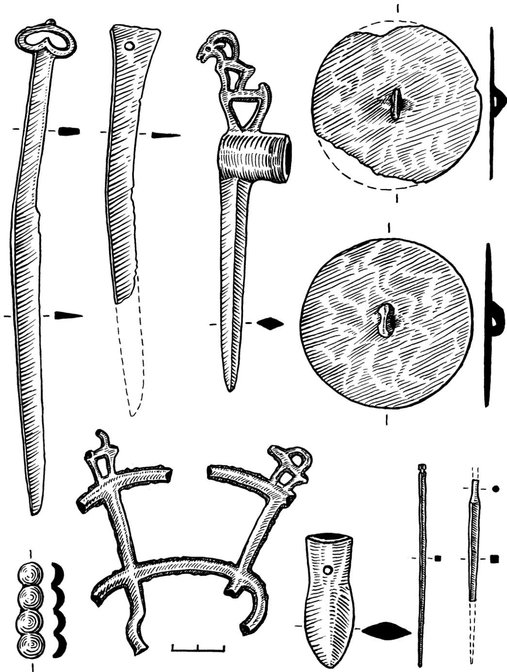
49. Курган Береш III. Могилы 2 и 3. Изделия из бронзы: 1-2. ножи; 3. чекан; 4-5. зеркала; 6. 4-частная бляшка; 6. штандарт; 7. вток; 8-9. шилья.
