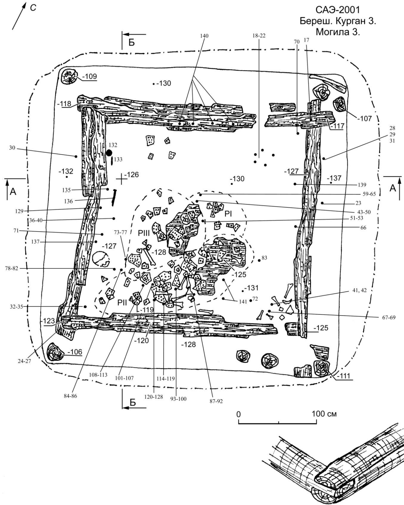
46. Курган Береш III. Могила 3. Дно. План.
