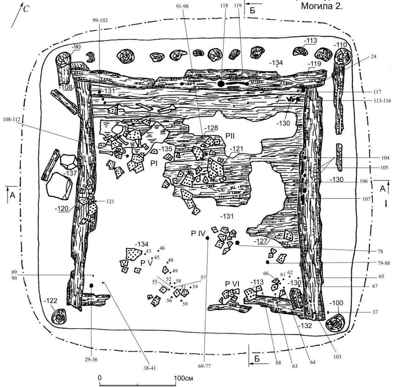
31. Курган Береш III. Могила 2. Дно. План.
