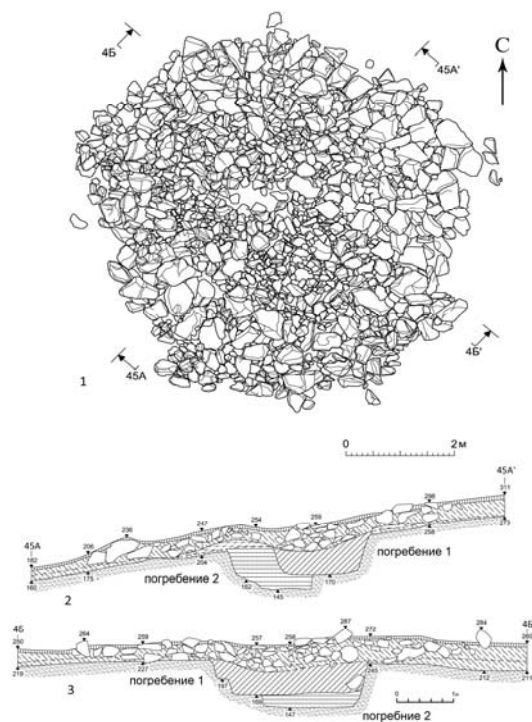
Рис. 3. План насыпи (1) и разрезы А–А', Б–Б' (2–3) кургана № 4
