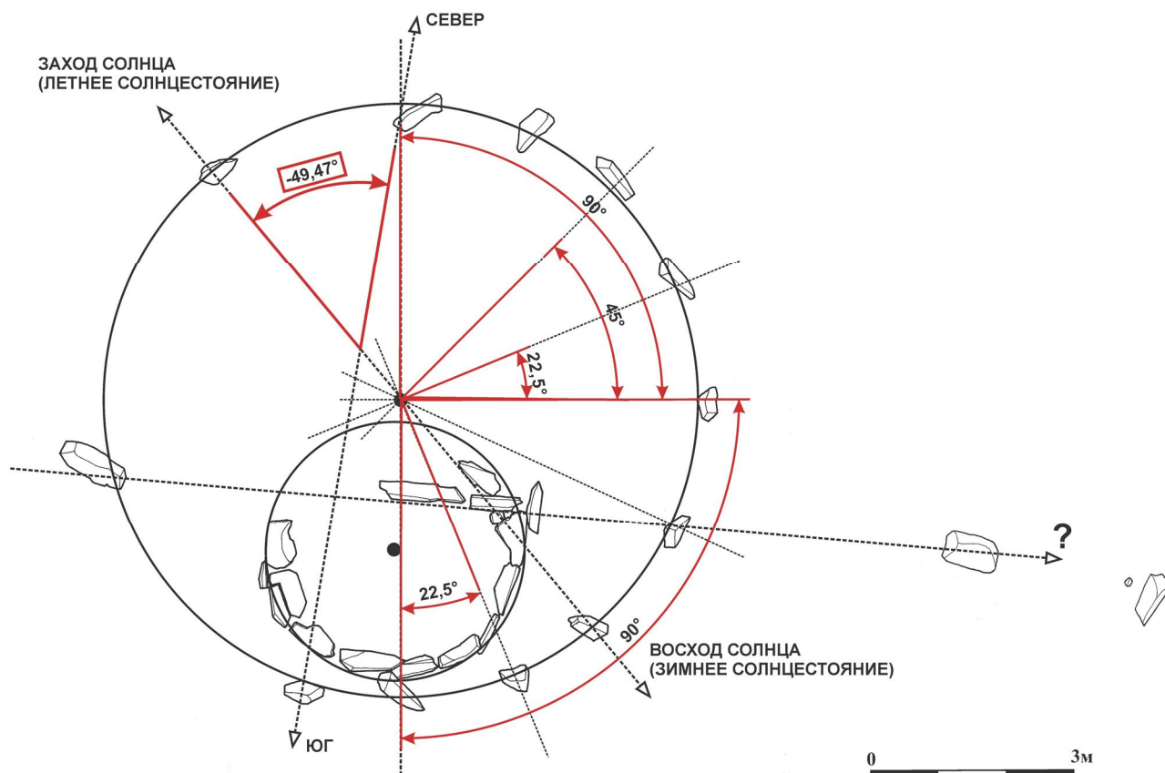
Рис. 20. Ограда Хух хушооны бом 1/4. Общий план Fig. 20. Ritual structure Khukh khushoony bom 1/4 (Zavkhan aimag, Mongolia). Plan
