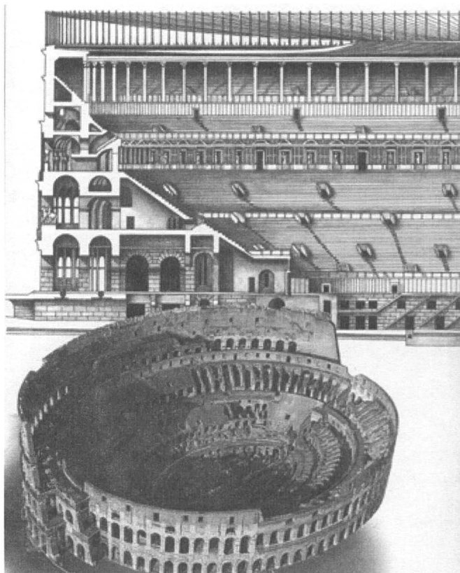
Рис. 23. Амфитеатр Флавиев (Колизей). Общий вид и разрез
