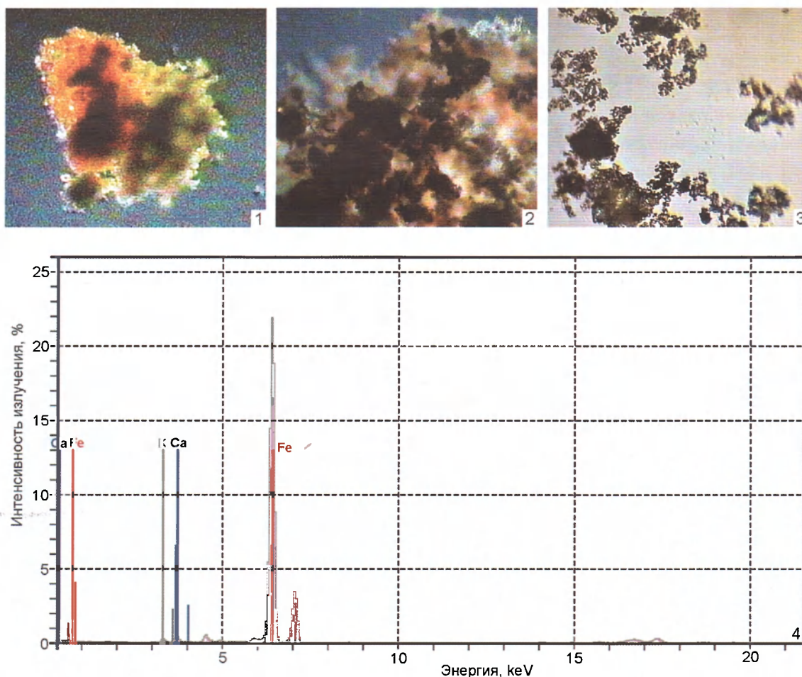
Рис. 4. Стоянка Ланино 1/8, галька с гравировкой: 1–3 — микрофотографии в полиполяризованном свете (1 — проба № 2, фрагмент красной краски; 2 — проба № 3, фрагмент желтой краски; 3 — проба № 5, содержимое водного экстракта из красной краски [органика]); 4 — спектр рентгеновской флуоресценции материала камня
