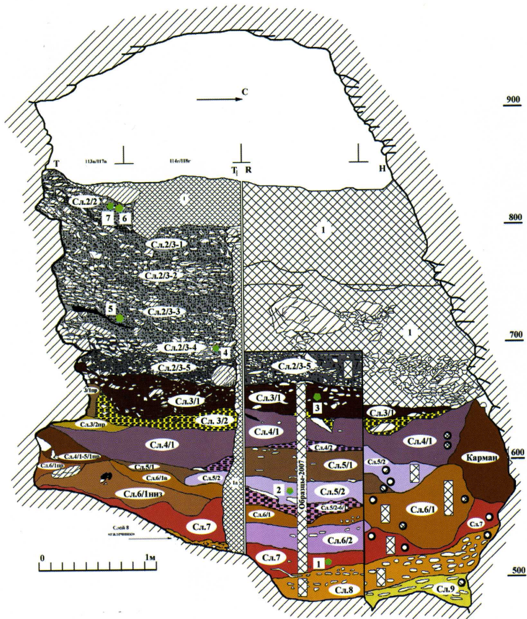
Рис. 1. К статье С.А. Кулаков, М.А. Кулькова: Предварительная корреляция результатов стратиграфического и литолого-минералогического изучения отложений Ахштырской пещерной стоянки. Обобщенный поперечный разрез пещерных отложений Т-Т 1 -R-H, 1996–2008 гг.
